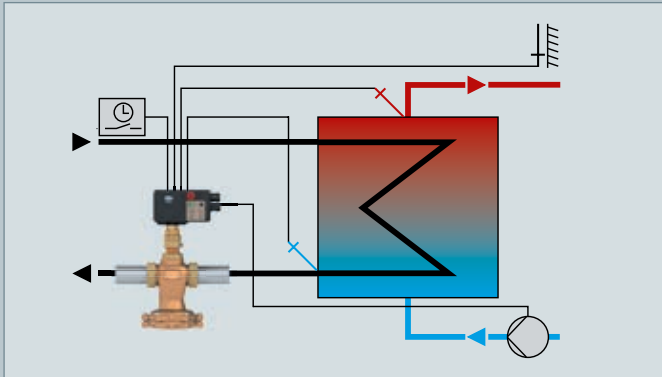
Regulacija temperature odvisna od temperature okolice in omejitve temperature povratka.
