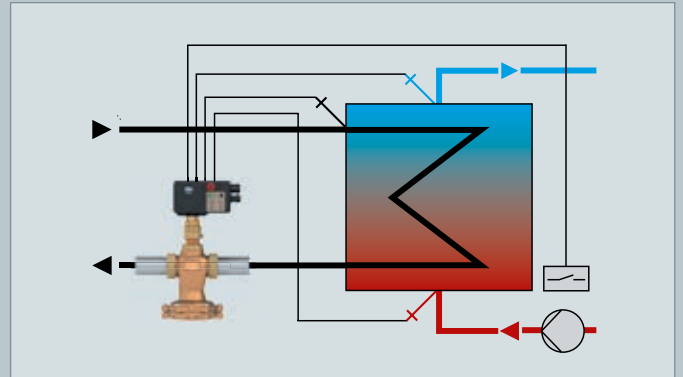
Regulacija temperature pretoka na sekundarju odvisna od omrežne temperature in temperature povratka na sekundarju.
